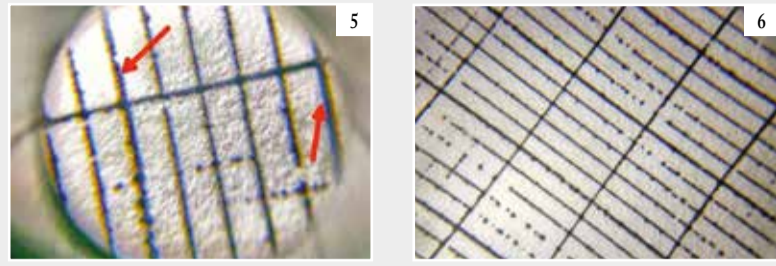
Fig. 5 : Aberrations chromatiques. On remarque le doublement par des lignes bleues. | Fig. 6 : Aberrations géométriques. Il y a une distorsion de l'image.
