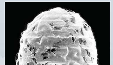
Pointe usagée Fabrication électrolytique
