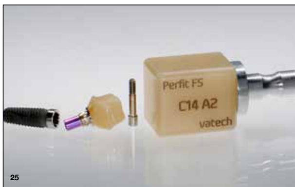
Slika 25 in 26: Dokončan nosilec iz cirkonijevega oksida, izdelan iz Perfit FS ML A2 (Vatech).
