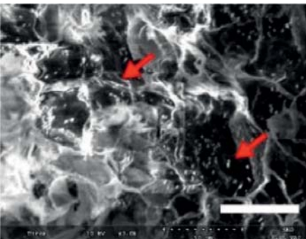
Microstructure de l'hydrogel de fibrine nanocomposite observée en microscopie électronique à balayage. Des nanoparticules sont indiquées par les flèches rouges. Barre blanche = 10 µm.
