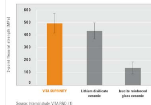
Рис. 2: После шлифования у образцов из VITA SUPRINITY наблюдается более высокая прочность при 3-точечном изгибе, чем у образцов из других керамических материалов. Источник: внутреннее исследование, VITA F&E
