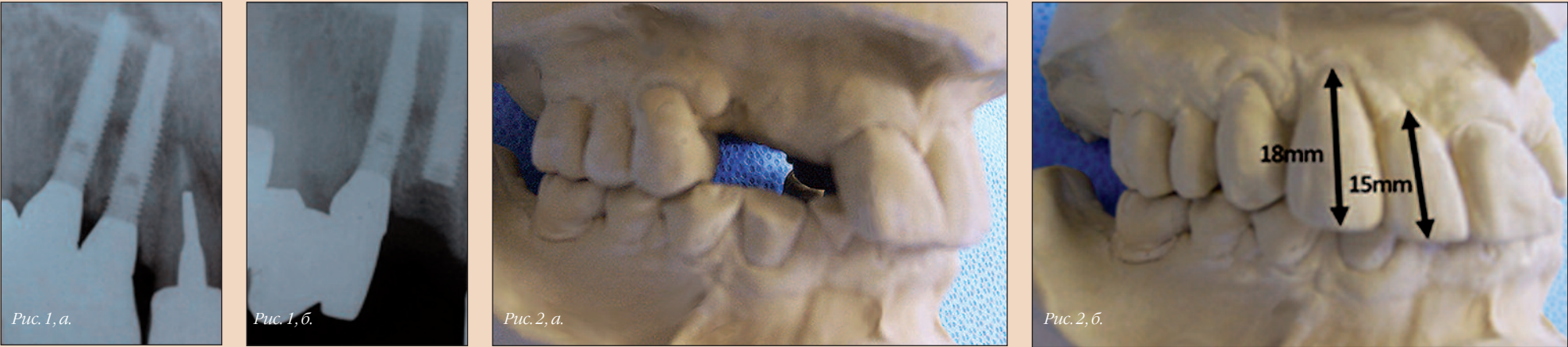
Рис. 1а, б. Имплантаты в области зубов 13 и 12 (Lifecore Bio-medical, 3,3×15 мм) до (а) и после (б) поломки. Рис. 2а, б. Ретроспективный анализ участка установки имплантатов 13 и 12 (а) выявил наличие существенного вертикального перекрытия, требующего постановки удлиненных коронок (б) для сохранения надлежащей эстетики, и одновременно – своеобразной окклюзии, ведущей к повышенной стираемости зубов.
