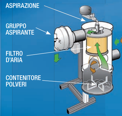
L'interno di un abbattitore di polveri per: sabbiatrice, box ritocchi, rapide e pulitrici
