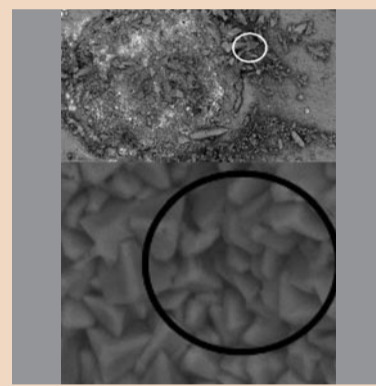
Рис. 1, г. Микроструктура цемента на основе ортофосфата кальция после отверждения. Механическая стабильность материала обеспечивается зацеплением молекул
