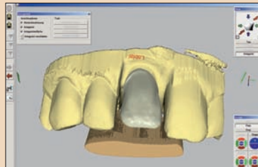
Şekil 5. CEREC 3 cihazında 3 boyutlu olarak oklüzon ayarlaması.
