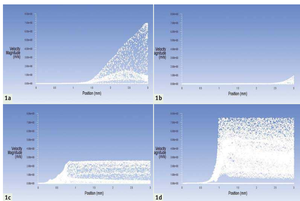
Figs. 1 a-d : intensité de la vitesse d'irrigation illustrant l'étendue de la zone morte. Pointe d'aiguille à extrémité ouverte (a) : la vitesse diminue progressivement à 1,5 mm de la région située apicalement par rapport à la pointe de l'aiguille. Pointe d'aiguille à fenêtre latérale (b) : la vitesse est nettement inférieure à celle observée avec l'aiguille à extrémité ouverte, et elle n'augmente que sur 0,5 mm. Irrigation par pression négative apicale (c) : une vitesse constante légèrement supérieure à celle de l'irrigation par aiguille à fenêtre latérale est observée et elle demeure constante dans le flux d'irrigant circulant en direction coronaire. Irrigation ultrasonique (d) : on observe la vitesse de plus forte intensité, constante jusqu'à au moins 3 mm de la région située coronairement par rapport à la position de la pointe de l'aiguille. 35
