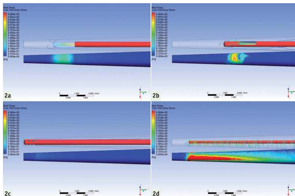
Figs. 2 a-d : distribution moyennée dans le temps de la contrainte de cisaillement pariétale illustrant une distribution plus uniforme sur la paroi canalaire dans le cas de la pointe d'aiguille à extrémité ouverte (a). Pointe d'aiguille à fenêtre latérale (b) : montre un niveau élevé de contrainte de cisaillement dans une région localisée alors qu'aucun niveau de contrainte n'est observable lors de l'irrigation par EndoVac (Kerr) ; c). L'irrigation ultrasonique (d) montre les niveaux les plus élevés de contrainte de cisaillement, distribués sur la plus grande surface de la paroi canalaire. 35
