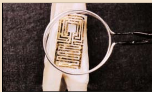
Ο αισθητήρας αποτελείται από ένα στρώμα γραφίτη εντυπωμένο σε ένα βιοαπορροφήσιμο υπόστρωμα μεταξίου
